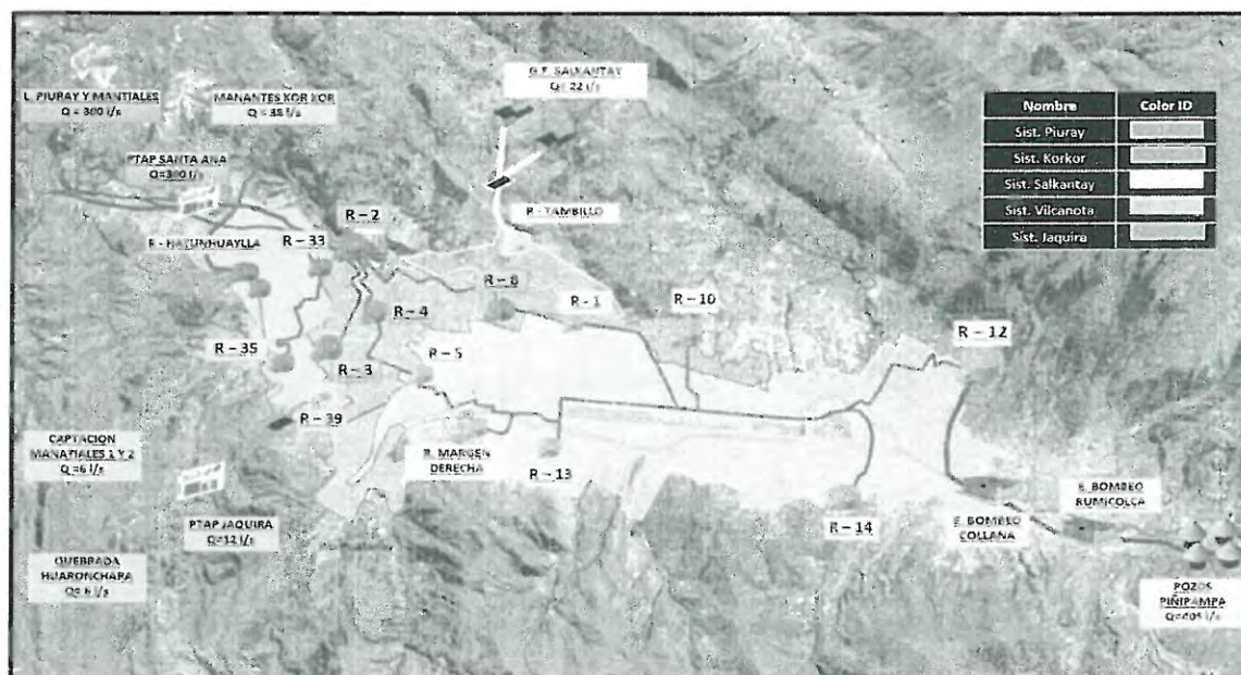
GRÁFICA N° 50: ESQUEMA GENERAL DEL SISTEMA DE AGUA POTABLE
